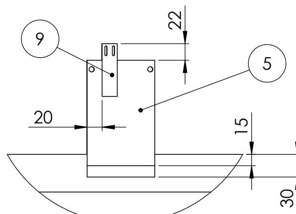
DÉTAIL A ECHELLE 1 : 5
